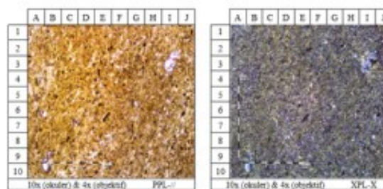
Gambar 13. Kenampakan sayatan tipis Batulempung dengan kode 03-Tma pada Formasi Air Benakat (Tma)
